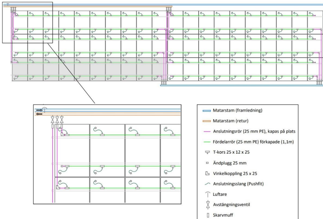
Bild 3, rörkoppling solhybrid
