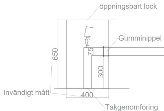
Bild 6, exempel takgenomföringshuv
