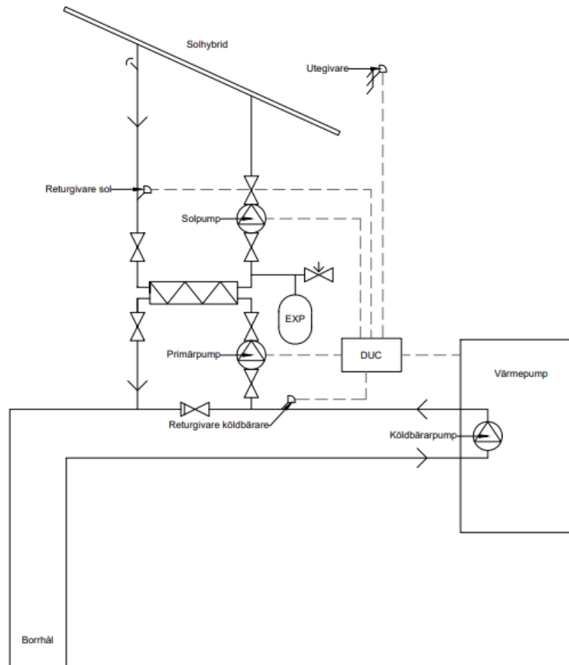
Bild 7, styrfunktion med DUC
