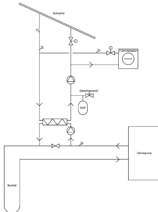
Bild 4, standardsystem med frånluftsåtervinning
